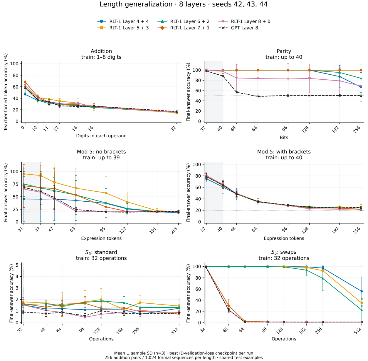
图 12 分布内最佳检查点的长度泛化，三个初始化种子。 加法在每种操作数位数的 256 对样本上测量教师强制答案 token 准确率；形式任务在每个长度的 1,024 条序列上测量最终标签或最终状态准确率。点与误差棒表示种子 42、43 和 44 的均值 ± 样本 SD，所有模型使用相同测试样本。SD 误差棒可能超出准确率范围。灰色区域表示训练长度，横向点线表示均匀预测准确率。无括号模五运算使用实际奇数表达式长度，不包含 BOS 和末尾等号。
