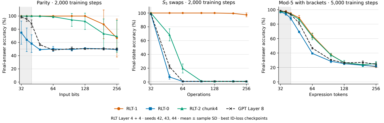
图 8 固定 4 + 4 配比下的反馈频率比较。 展示 RLT-1 ( B = 1 )、RLT-2 chunk4 ( B = 4 )、RLT-0 ( B = \infty ) 和 GPT Layer 8 在全部原生测试长度上的最终答案或状态准确率。奇偶校验与交换 S_5 训练 2,000 步，带括号模五训练 5,000 步。所有模型均使用种子 42–44 及其最低 ID 损失检查点。误差棒为未经裁剪的样本 SD，灰色区域标记训练长度，虚线标记均匀预测参考值。
