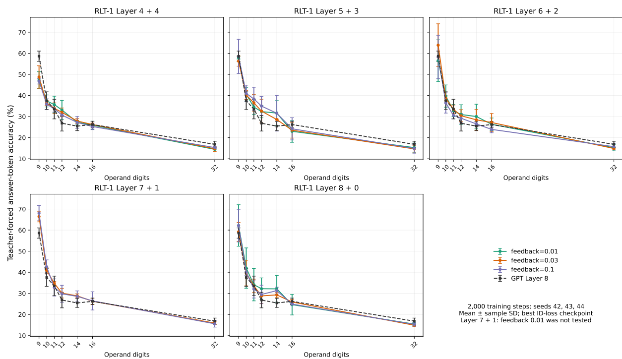
图 28 不同反馈系数下的加法泛化。 每个子图固定一种 RLT-1 配比，比较已测试的反馈系数与 GPT Layer 8；7 + 1 未测试 \alpha = 0.01 。点和误差棒表示种子 42、43、44 的均值 \pm 样本标准差；所有模型训练 2,000 步，学习率调度相同。准确率为教师强制答案 token 准确率，每个长度共用 256 个样本。
