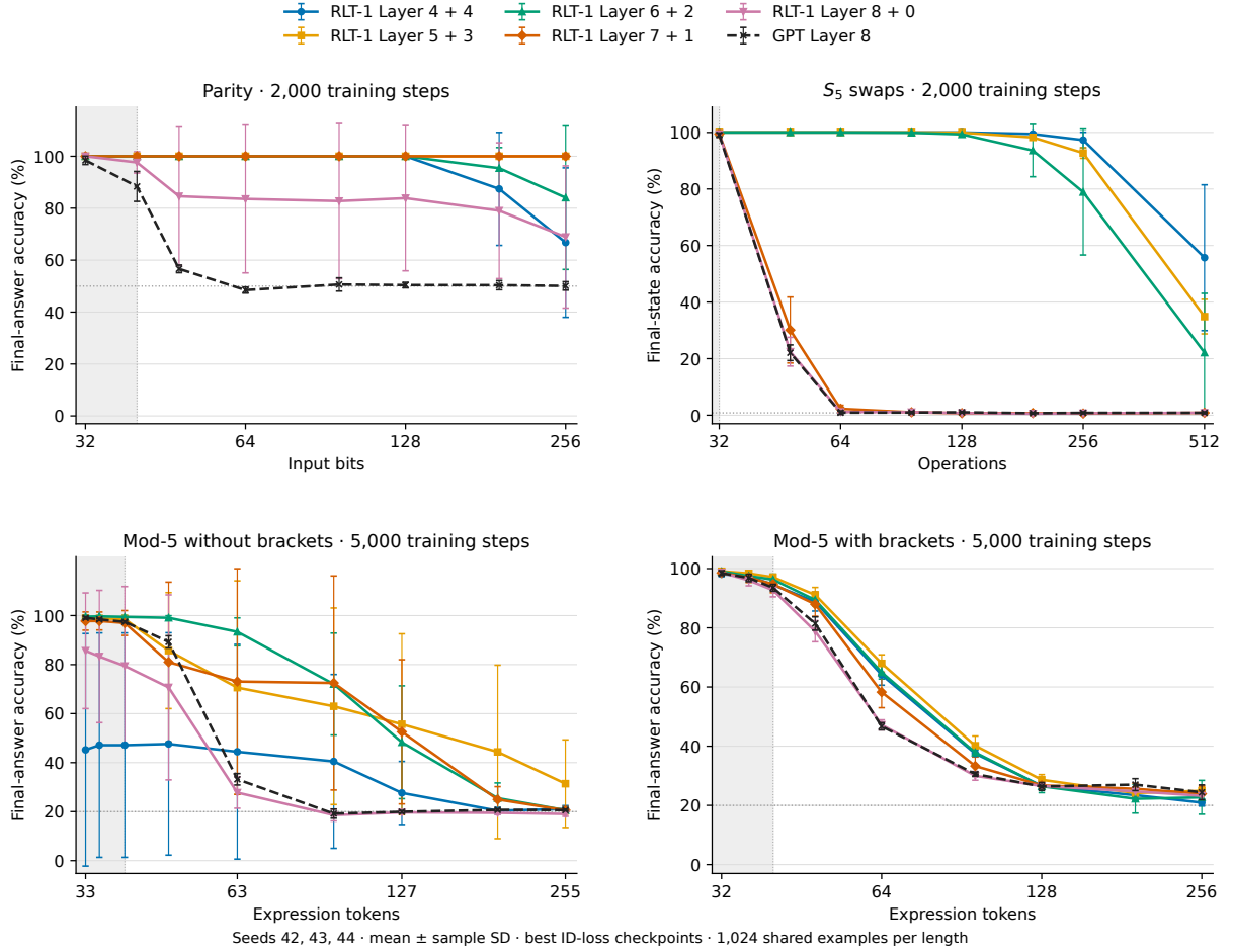
图 6 不同编码器与解码器配比的长度泛化。 五种 RLT-1 配比与 GPT Layer 8 均展示完整测试长度网格。上排的奇偶校验与交换 S_5 使用 2,000 步训练结果；下排模五任务的所有模型均训练 5,000 步。各次运行选择最低 ID 损失检查点，同分时取最早一步。点与未裁剪的误差棒表示种子 42、43、44 的均值 \pm 样本 SD，每种长度使用相同的 1,024 个样本。灰色区域标记训练长度，水平虚线标记均匀预测准确率。无括号模五标注实际奇数表达式长度。完整的六任务 2,000 步对照见图 12。
