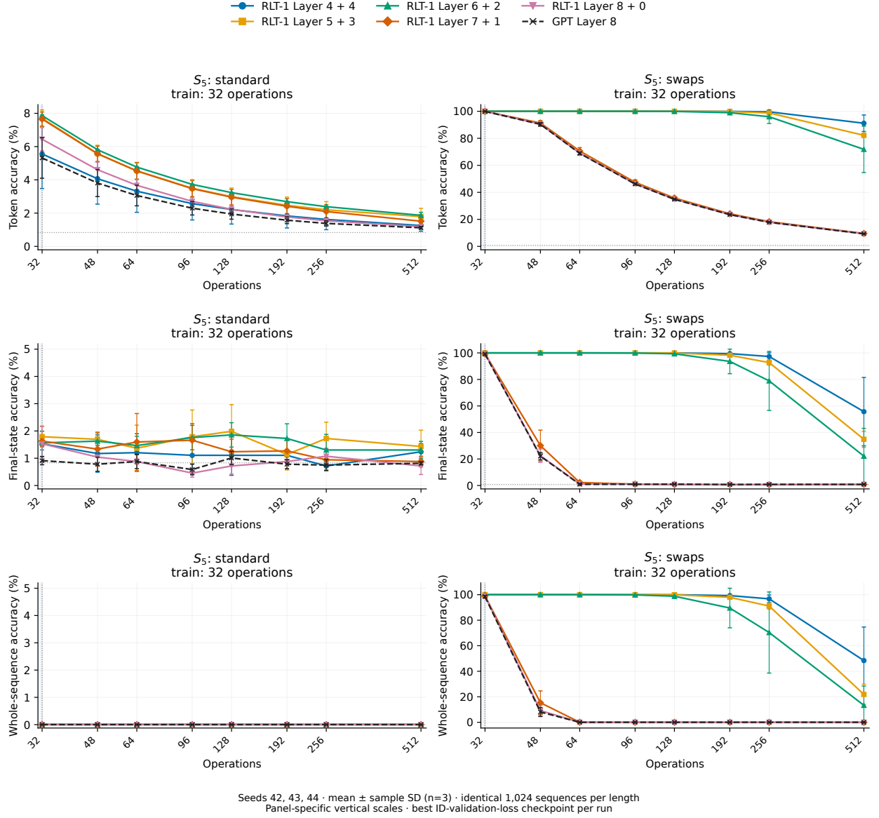
图 13 三种评分规则下的 S_5 长度泛化。各行依次为前缀 token、最终状态和全序列准确率，各列为标准与交换输入。每个模型与种子在每种长度下接收相同的 1,024 条序列。点和误差棒表示三个初始化种子的均值 ± 样本 SD。全序列成功要求所有前缀预测正确，各面板独立设置纵轴范围以展示标准 S_5 上较低的准确率。
